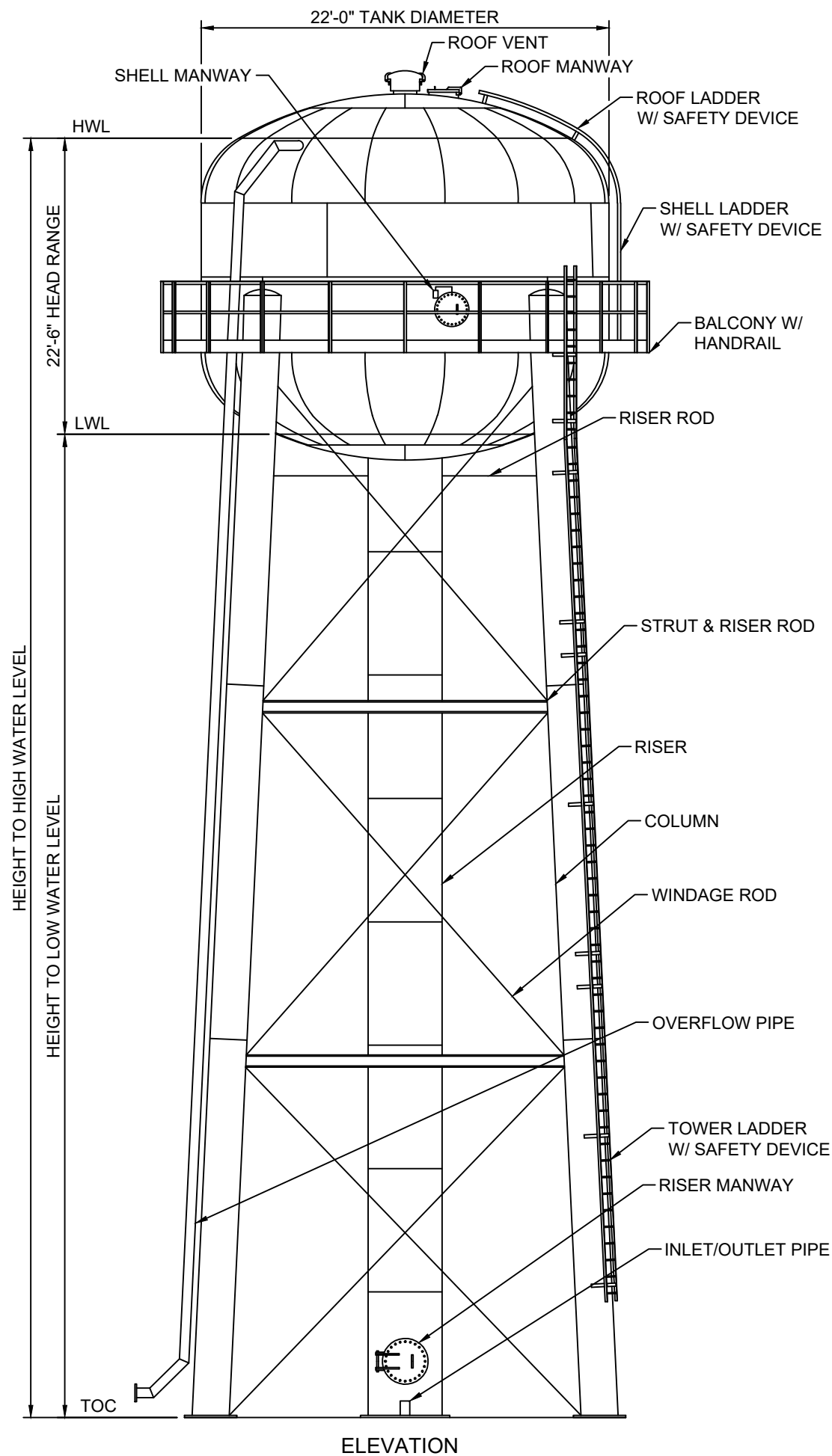
ELEVATION
