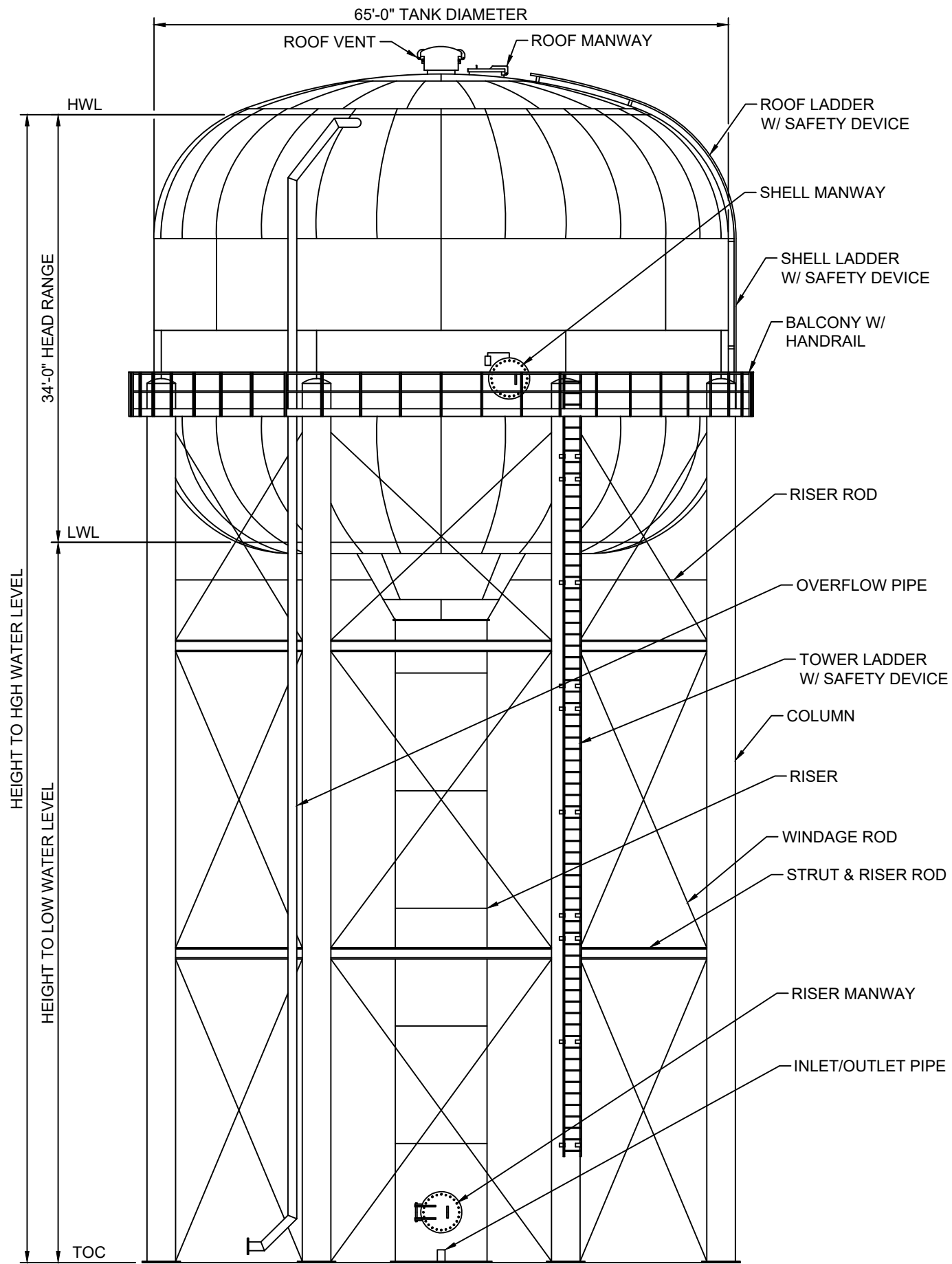
ELEVATION
