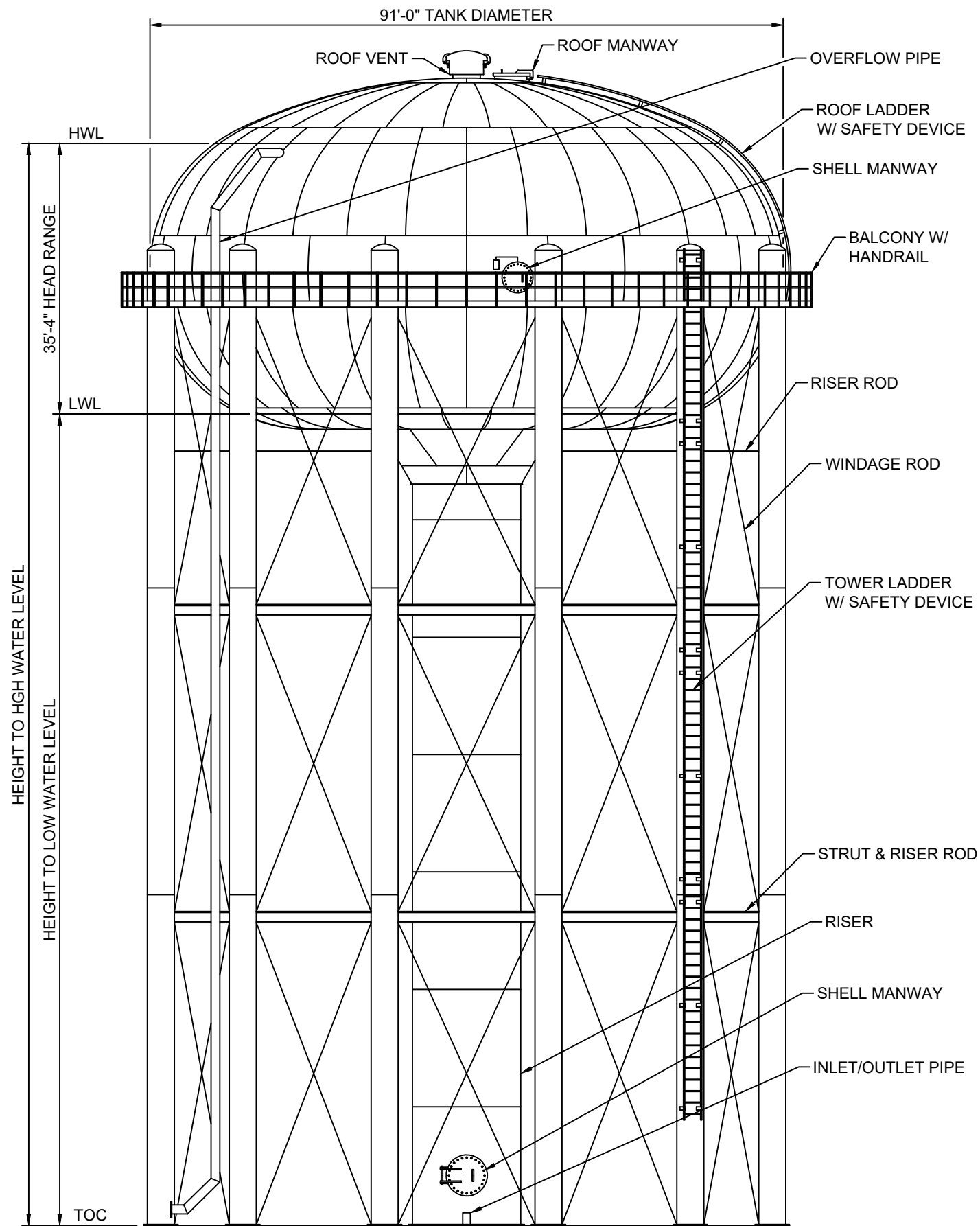
ELEVATION
