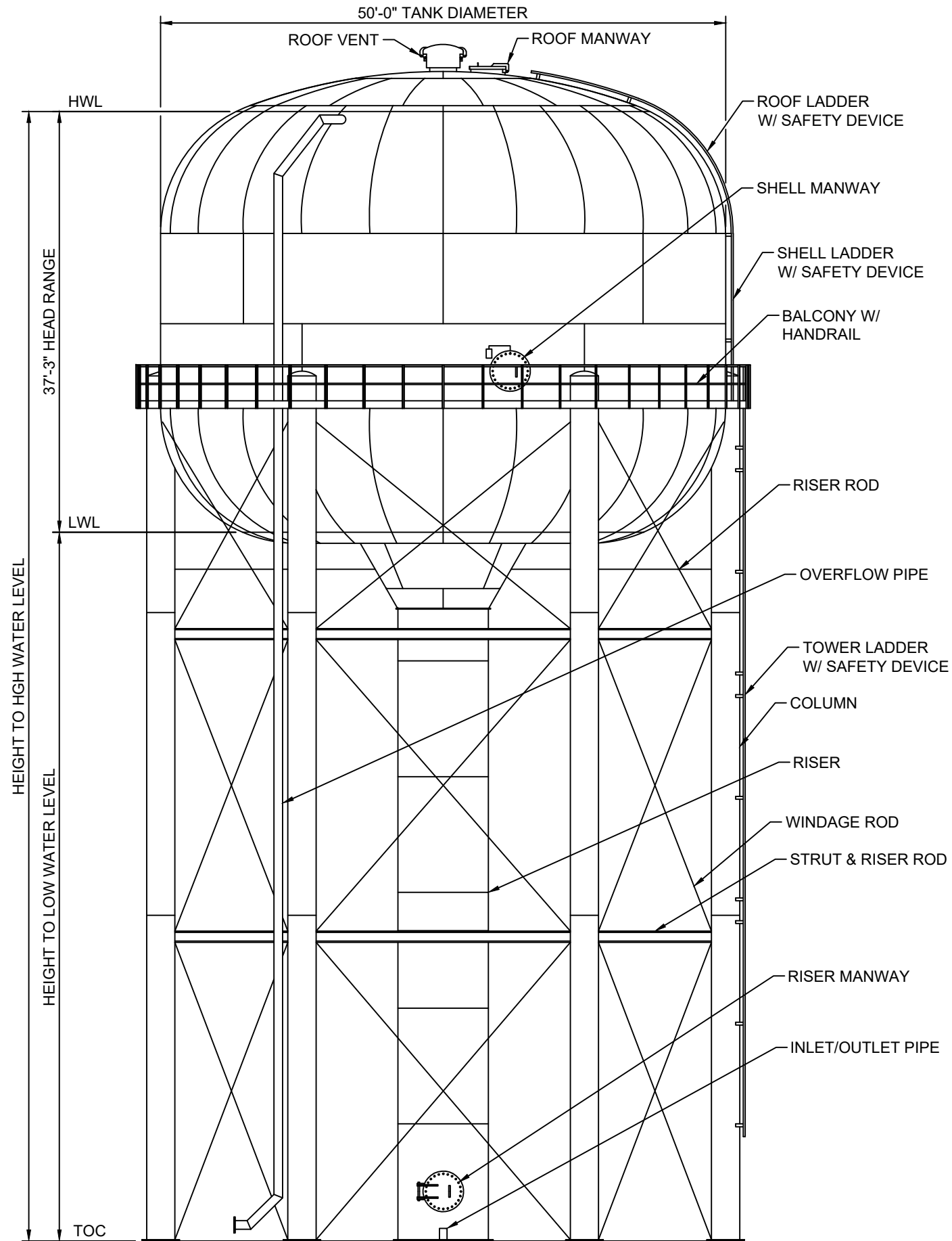
ELEVATION
