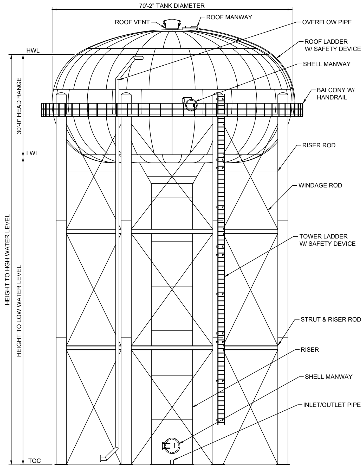
ELEVATION
